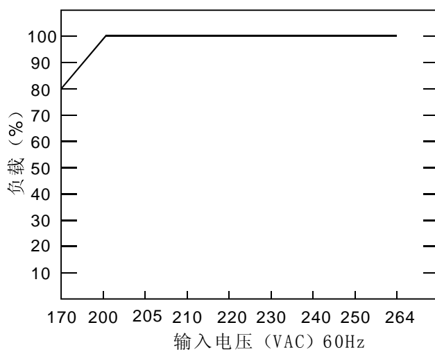
■ 输入降额曲线
