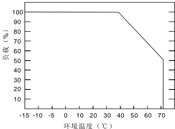
■ 温度降额曲线
